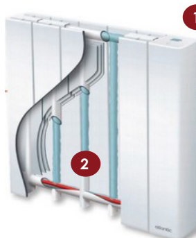
1 - Boîtier de commande digital 2 - Fluide thermoconducteur
